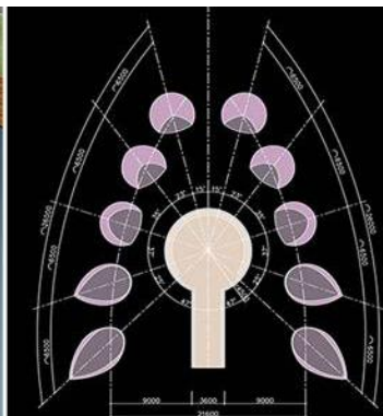
MẶT BẰNG CỤM BIỂU TƯỢNG
