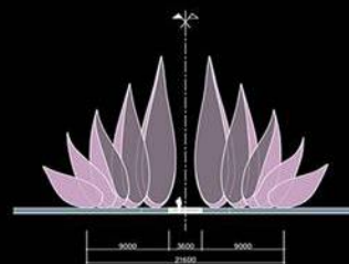
MẶT ĐỨNG CHÍNH CỤM BIỂU TƯỢNG
